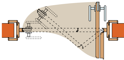
Schwenkbereich Triplan
